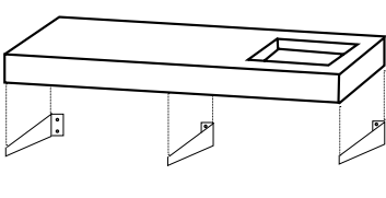
Geïntegreerde wastafel met skirts, vrijhangend met ophangbeugels
