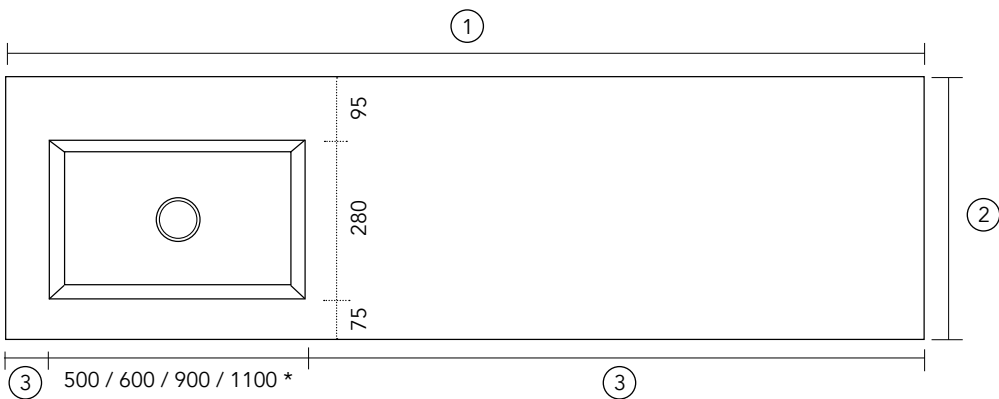
Geïntegreerde wastafel met skirts en onderkast
